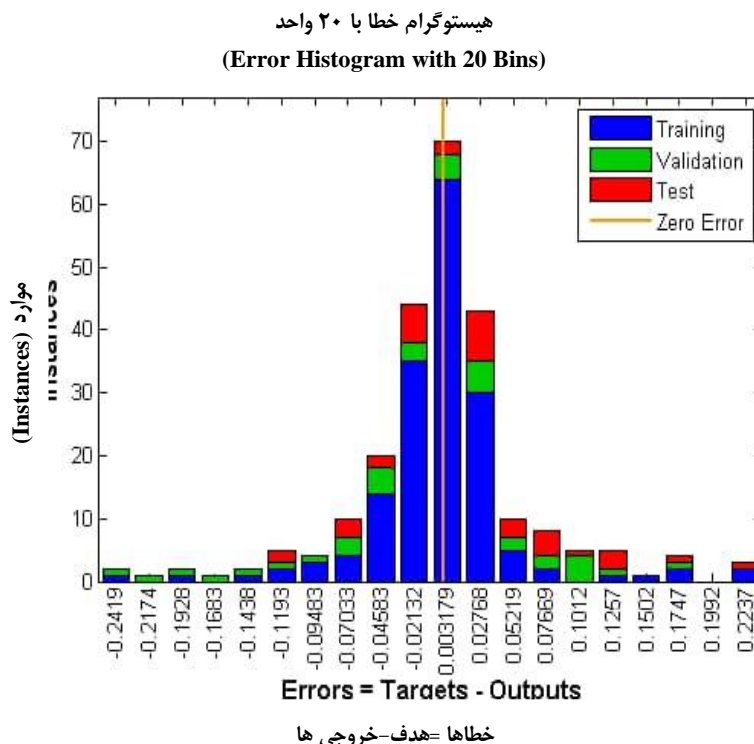
شکل ۳- نمودار هیستوگرام
